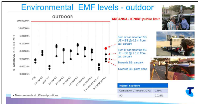
[그림 8] 실외 전자기장 환경
