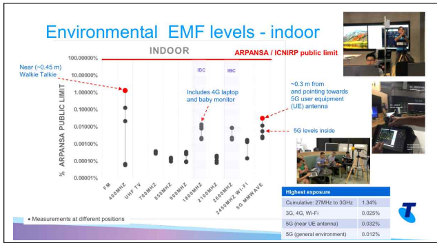
[그림 7] 실내 전자기장 환경
