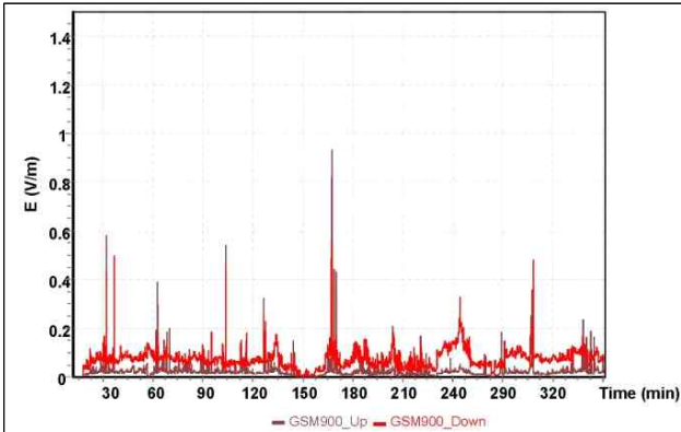
[그림 14] 비행 시 GSM900 시스템의 전자 장비 전자기장 강도
