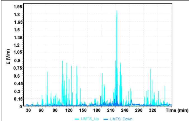
[그림 16] 비행 시 UMTS 시스템의 전자장비 전자기장 강도
