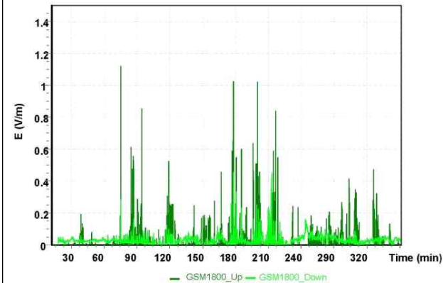
[그림 15] 비행 시 GSM1800 시스템의 전자 장비 전자기장 강도
