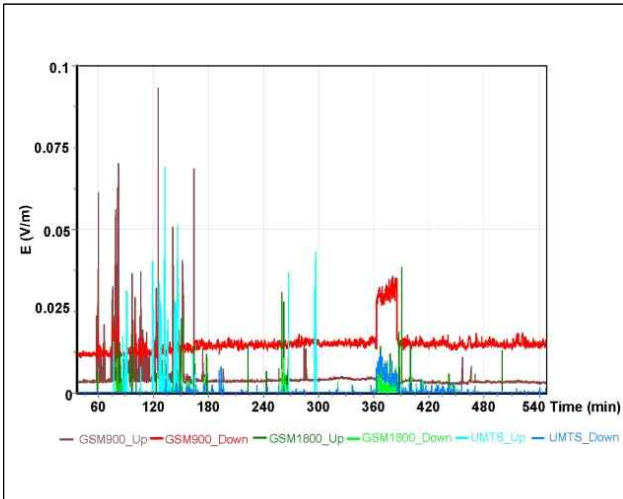
[그림 2] 관제탑에서 측정된 고주파 전기장 강도
