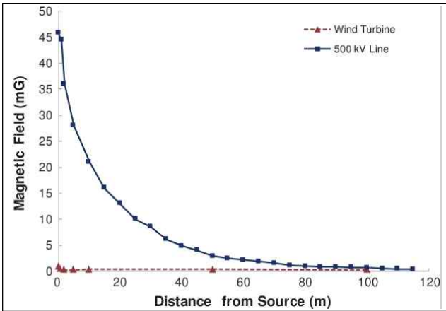
[그림 4] 풍력발전기와 500kV 송전선로에서의 자기장 값 비교
