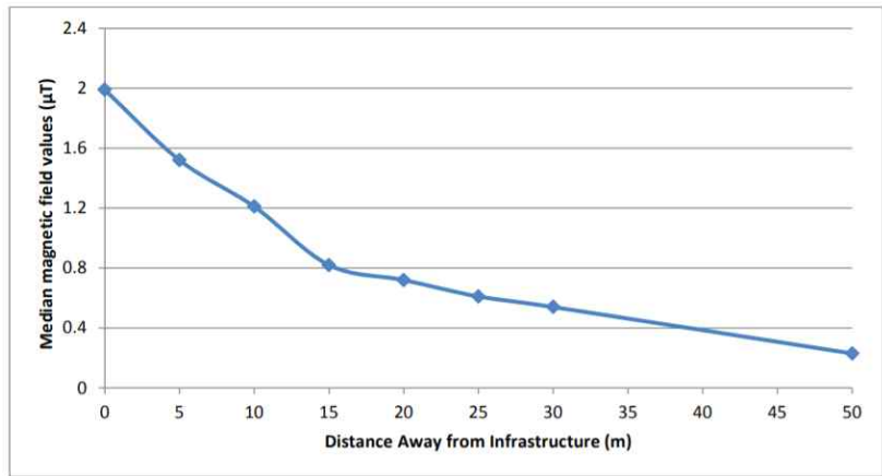
[그림 5] 거리에 따른 송전선로의 자기장 분포 (중위값)
