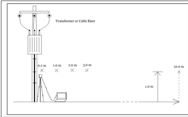
[그림 2] 주상 변압기, 입상주 측정 방법
