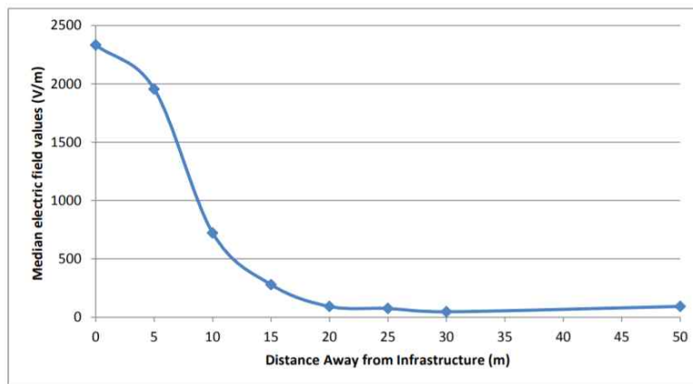
[그림 4] 거리에 따른 송전선로의 전기장 분포 (중위값)
