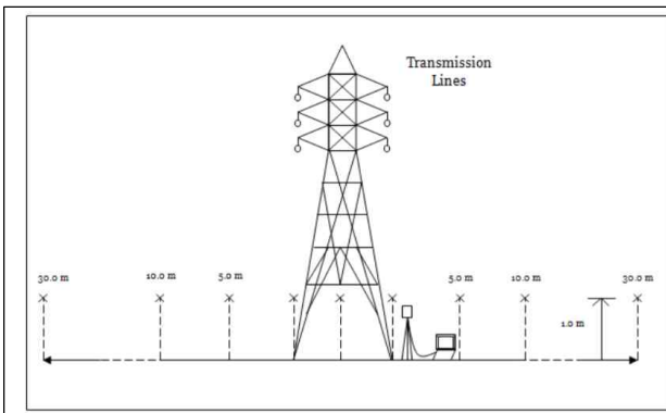
[그림 3] 송전선로 측정 방법
