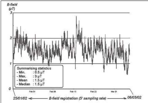
[그림 3] 380 kV 가공 송전선로의 시간별 자계강도
