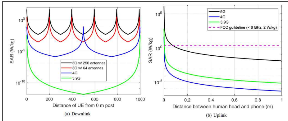
[그림 1] 다운링크와 업링크의 무선기술간 SAR 비교
